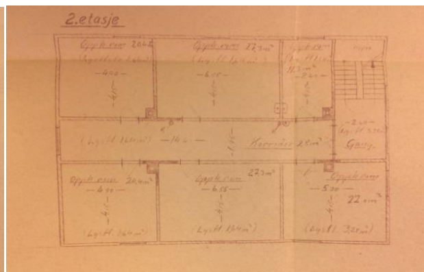
Plantegninger kasernebygg 1947, PBEs arkiv.
